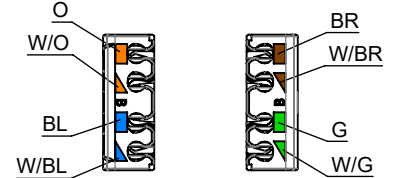
Anschlussbelegung / PIN assignment T568B nach / according to TIA-568.2-D
