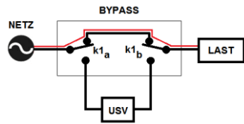
Abb. 15-2 Bypass-Betrieb
