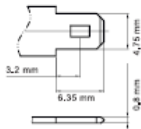
Polausführung S-4.8
